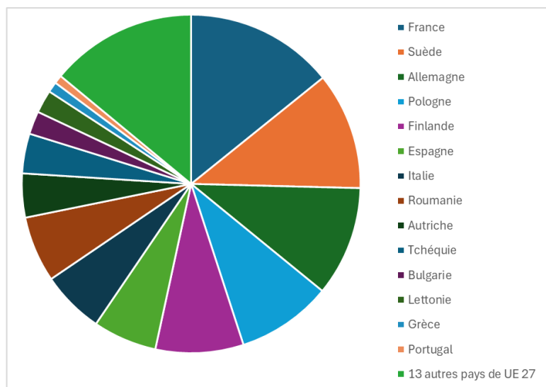
Figure 1. Répartition du stock (partie aérienne des arbres sur pied) des forêts dans les pays de l'UE des 27 (adapté de (7) )
